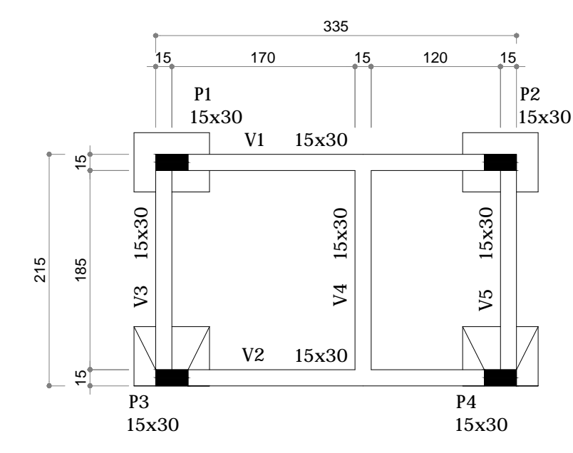
FORMA DO BALDRAME 1:50
