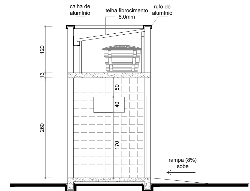
CORTE A A 1:50
