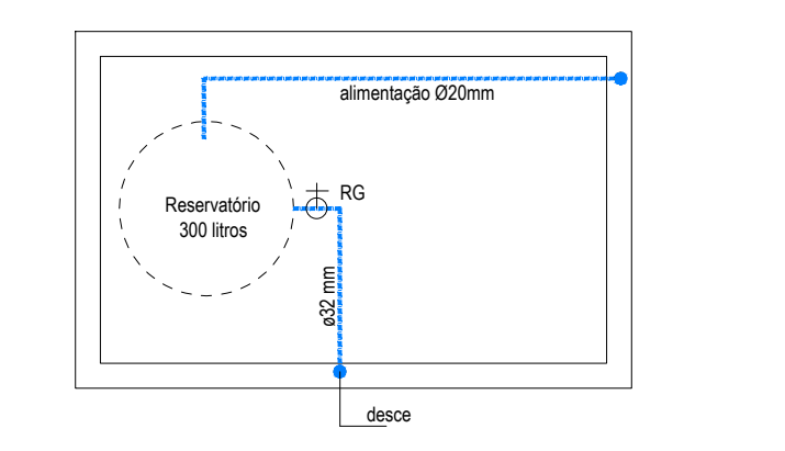
RESERVATÓRIO 1:50
