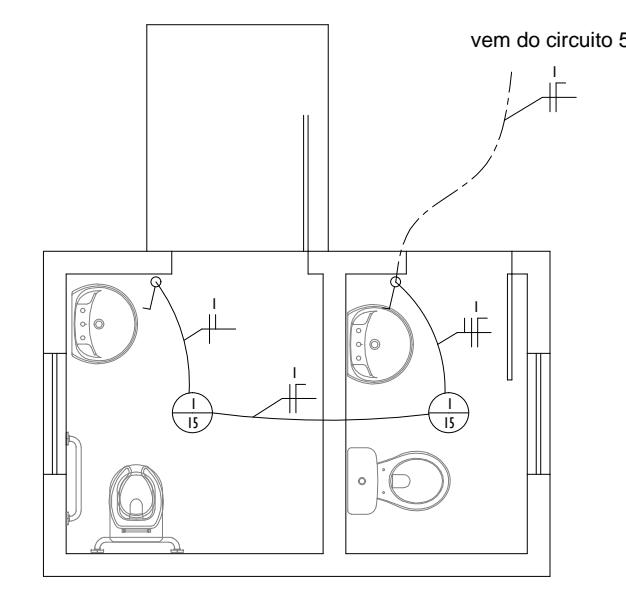
ELÉTRICO 1:50
