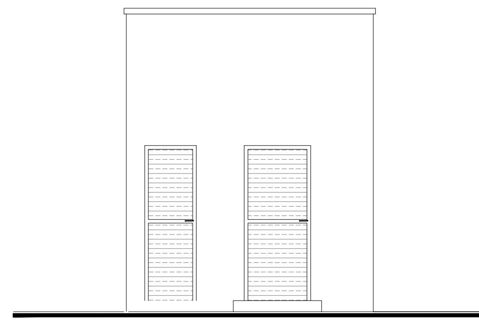
FACHADA FRONTAL 1:50
