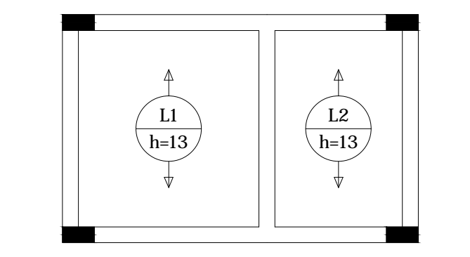
LAJE PRÉ-MOLDADA DE FORRO 1:50
