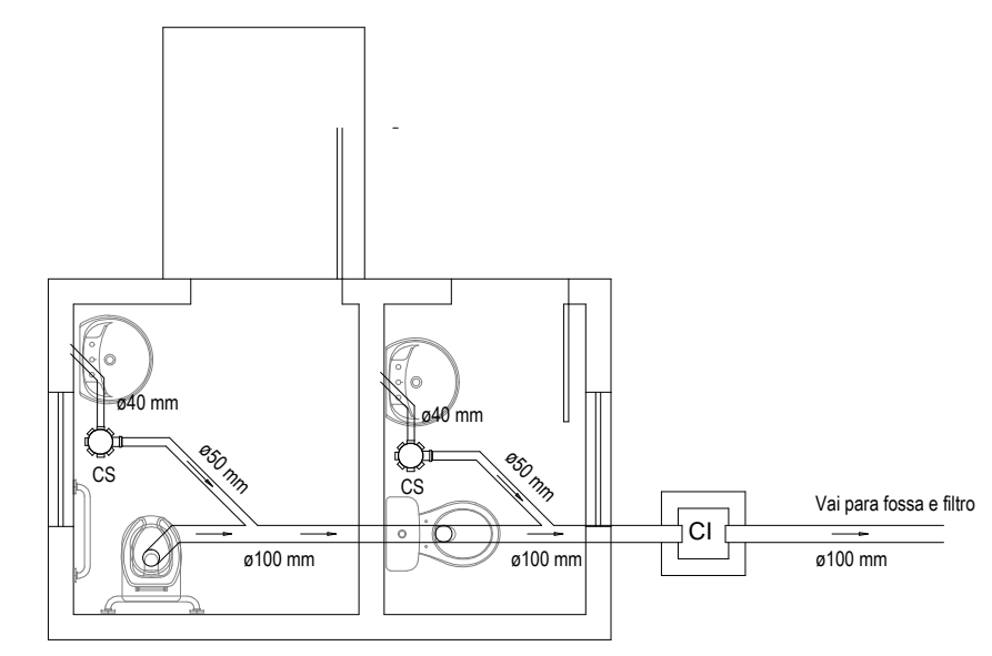
SANITÁRIO 1:50
