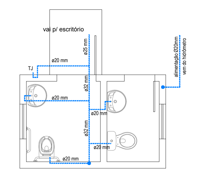
HIDRÁULICO 1:50
