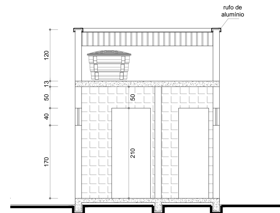
CORTE B B 1:50
