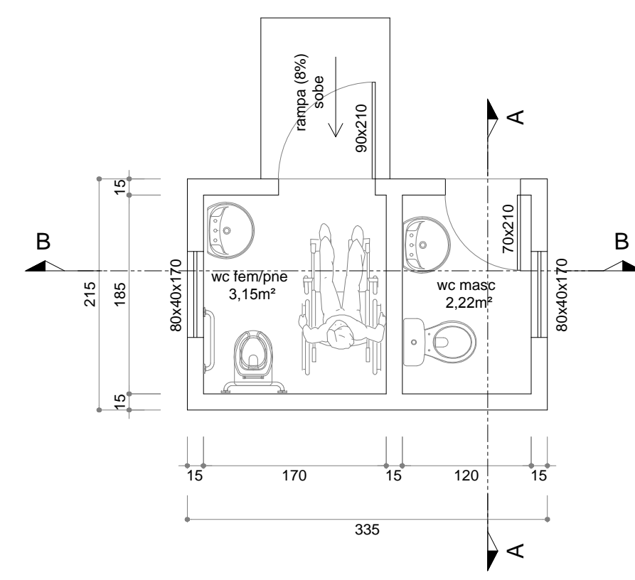
PLANTA BAIXA 1:50
