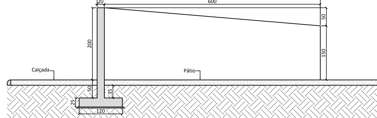
DEPÓSITO DE MATERIAIS CORTE "H-H" Escala 1:50
