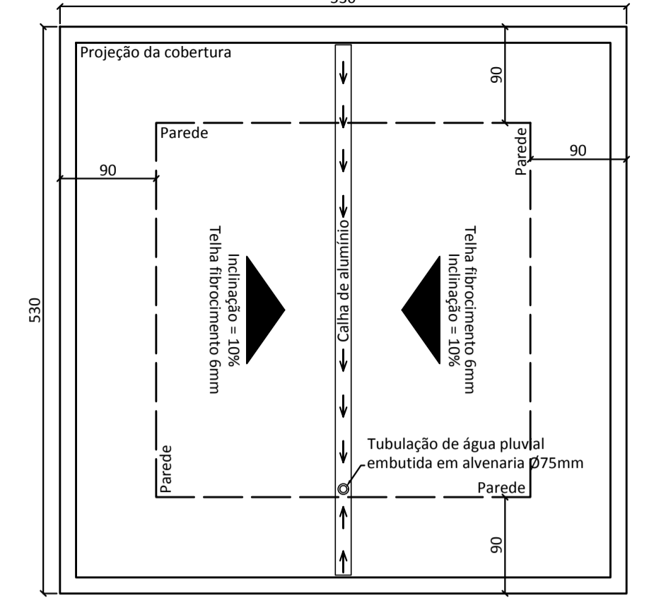
GUARITA PROJEÇÃO DA COBERTURA Escala 1:50
