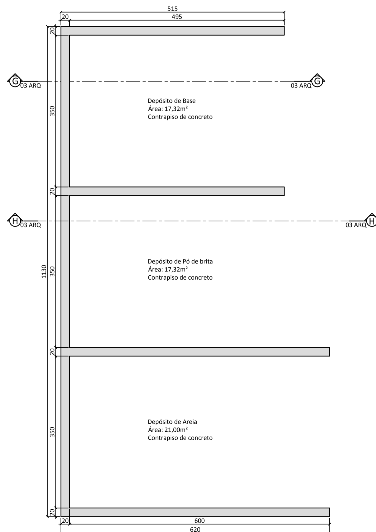
DEPÓSITO DE MATERIAIS - 62,29m² PLANTA BAIXA Escala 1:50
