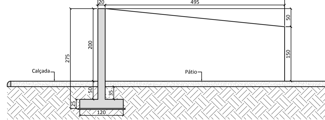
DEPÓSITO DE MATERIAIS CORTE "G-G" Escala 1:50
