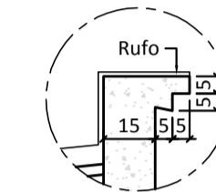
DETALHE "A" Escala 1:20
