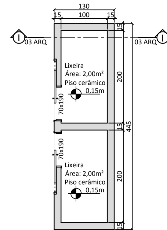
LIXEIRA - 5,78m² PLANTA BAIXA Escala 1:50
