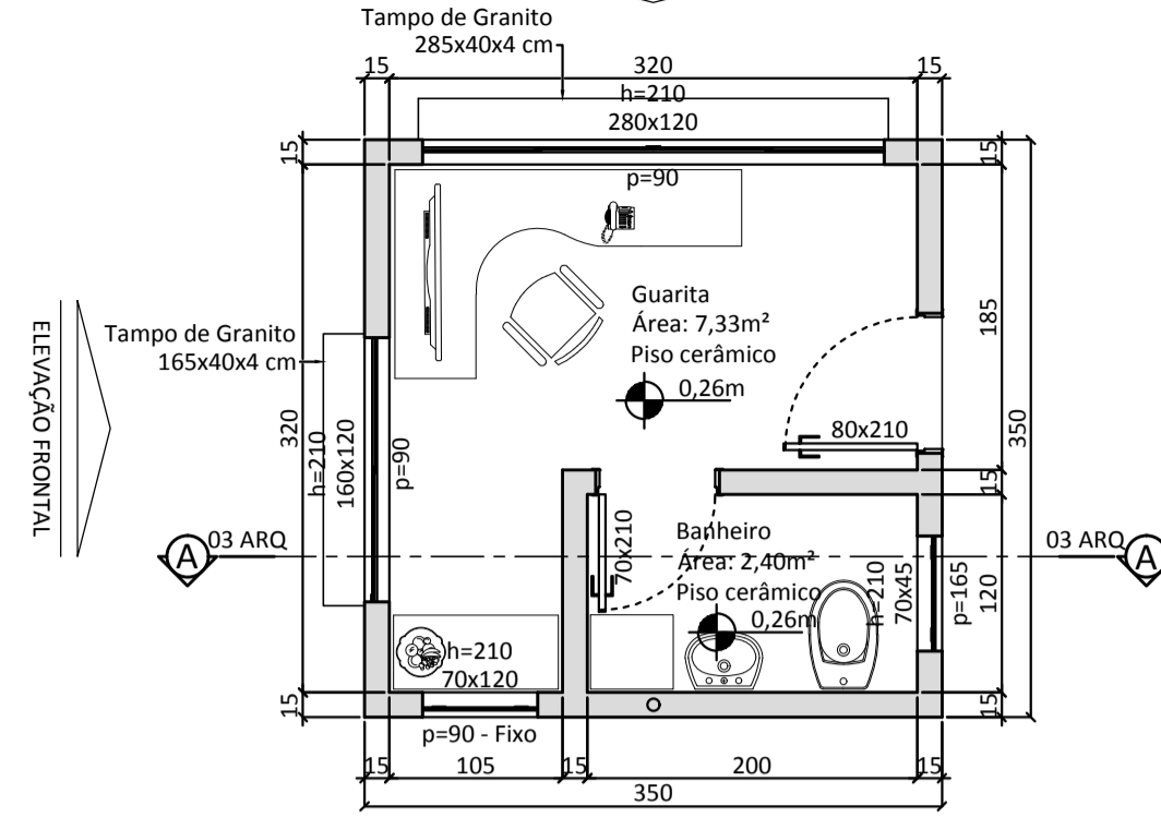
GUARITA - 12,25m² PLANTA BAIXA Escala 1:50
