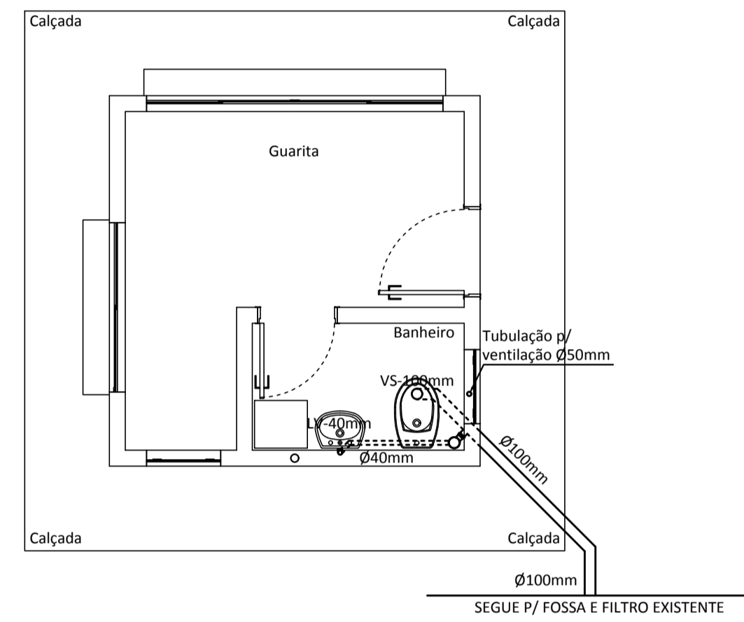
GUARITA DISTRIBUIÇÃO SANITÁRIA Escala 1:50
