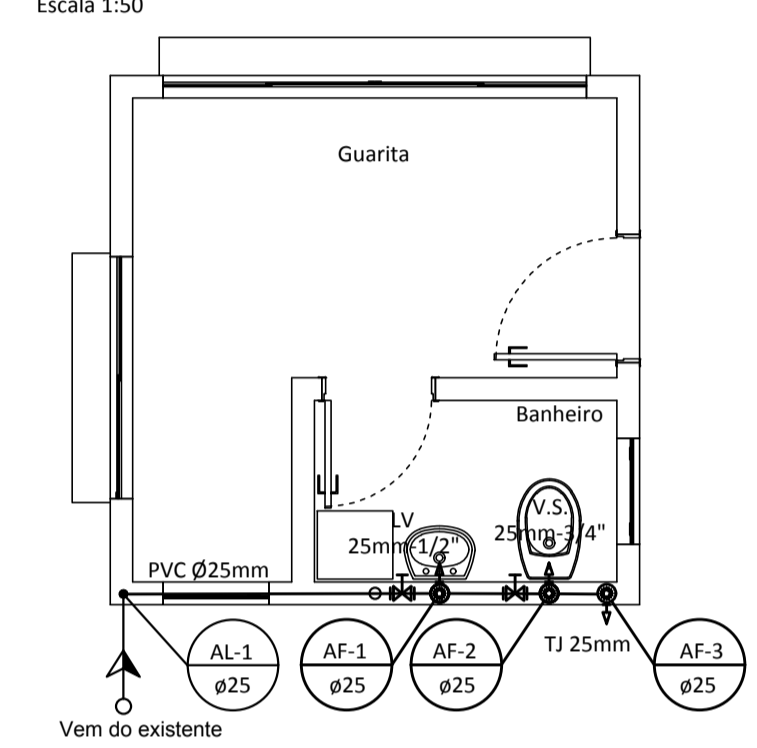
GUARITA DISTRIBUIÇÃO HIDRÁULICA Escala 1:50
