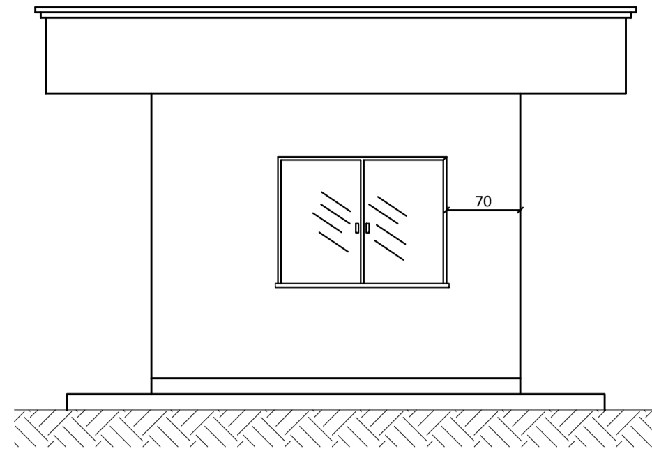
GUARITA ELEVÇÃO FRONTAL Escala 1:50
