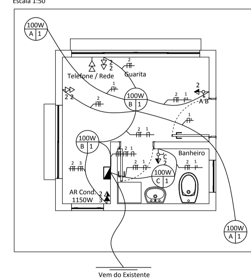
GUARITA DISTRIBUIÇÃO ELÉTRICA Escala 1:50
