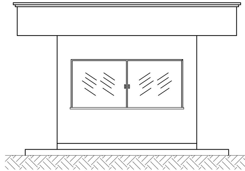
GUARITA ELEVÇÃO LATERAL Escala 1:50
