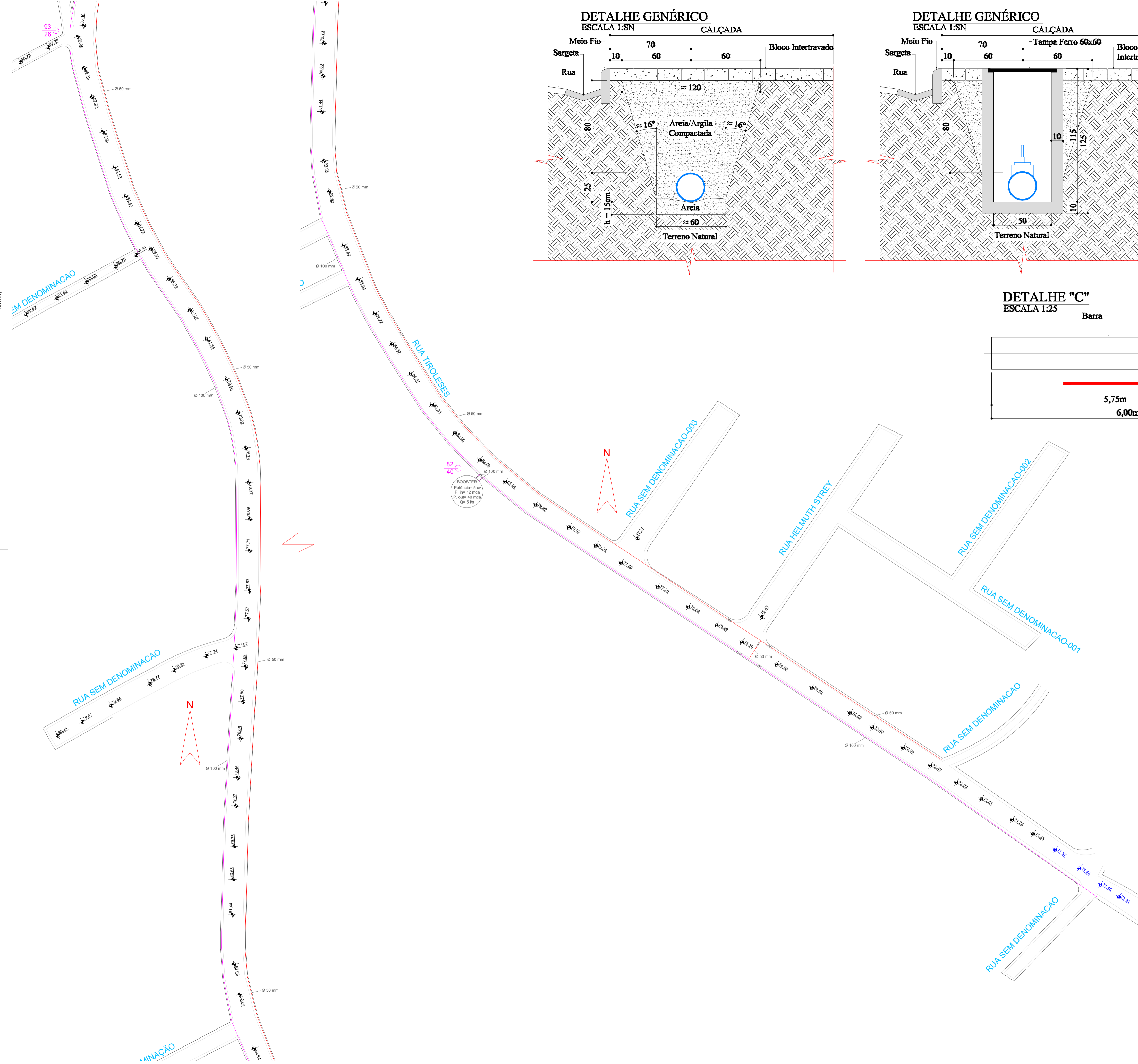
PLANTA BAIXA - REDE DE ADUÇÃO E DISTRIBUIÇÃO ESCALA: 1:1000
