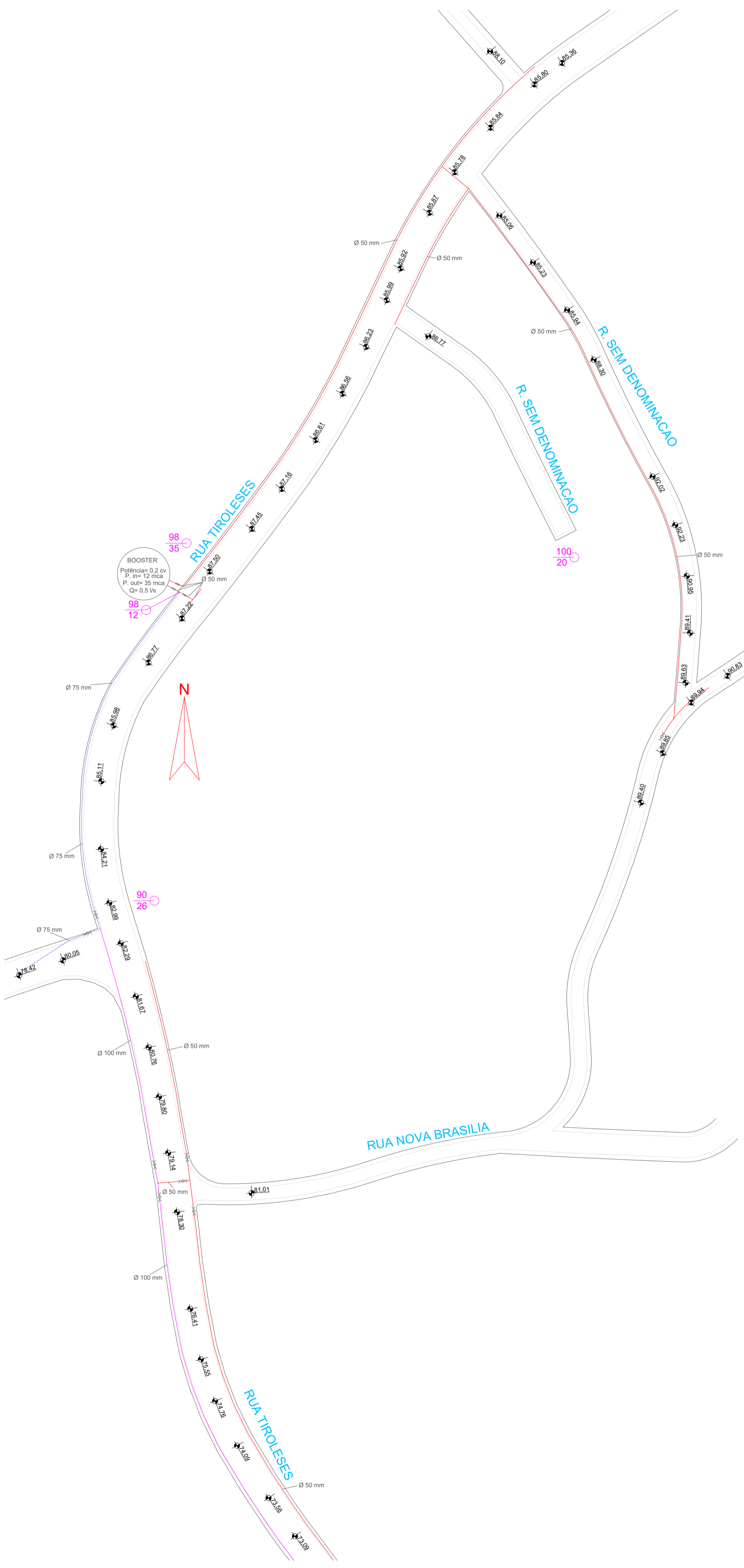
PLANTA BAIXA - REDE DE ADUÇÃO E DISTRIBUIÇÃO ESCALA: 1:1000
